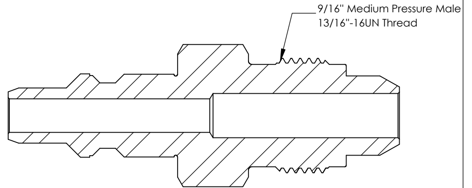
SECTION A-A
